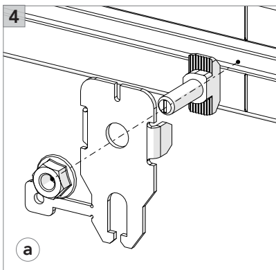
Innvendig beslag på Hub bæreprofil.
